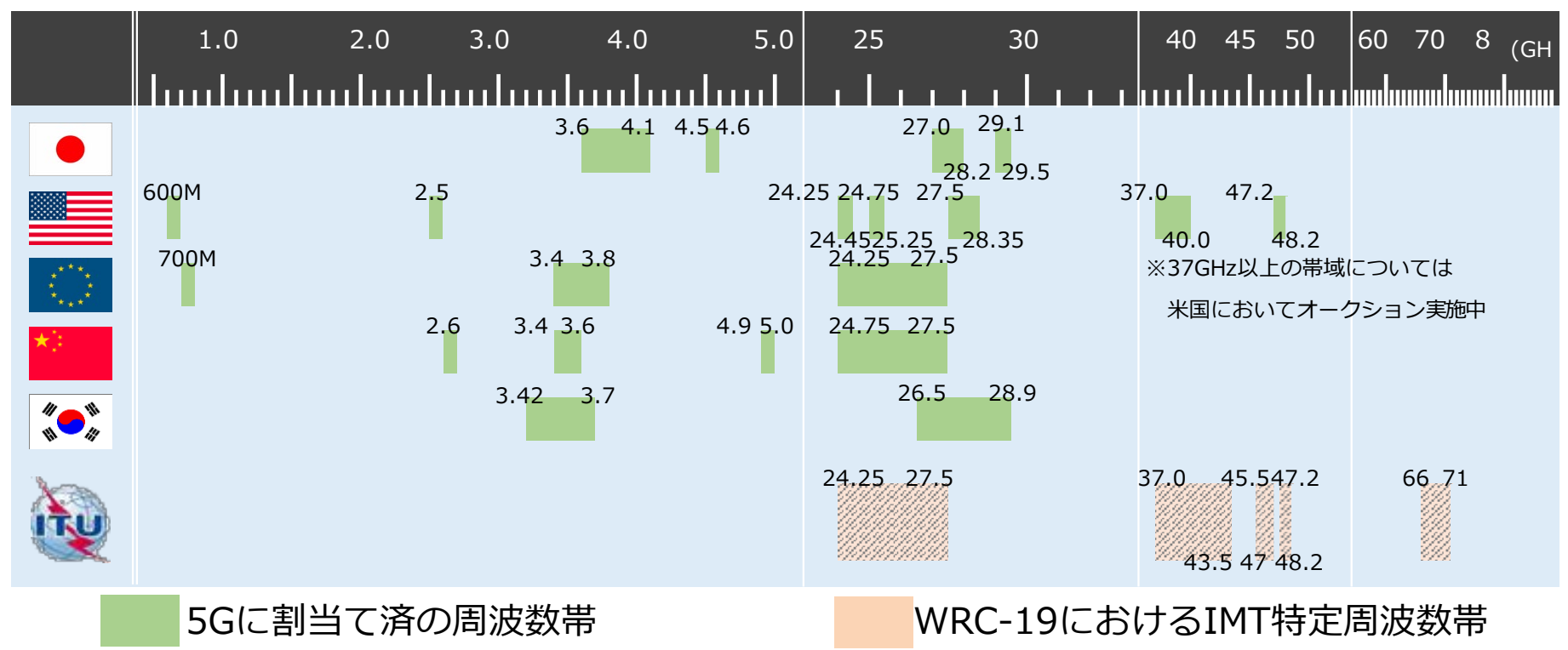
【各国のIMT-2020(5G)用周波数と議題1.13 IMT-2020用周波数特定の結果】
