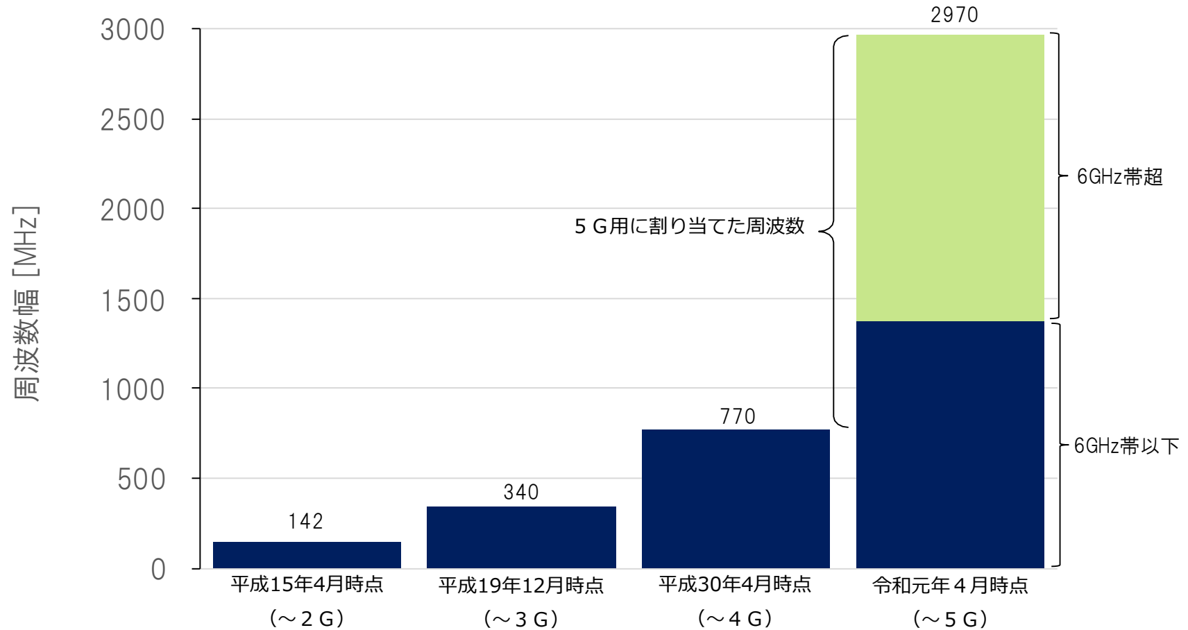
5G等に割り当てられた周波数の幅(合計)の推移
